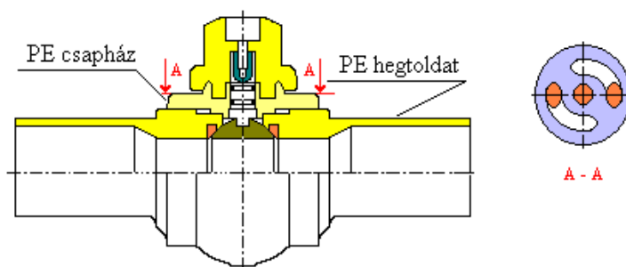
Hegtoldatos gömbcsap minta ábra (RMA)
