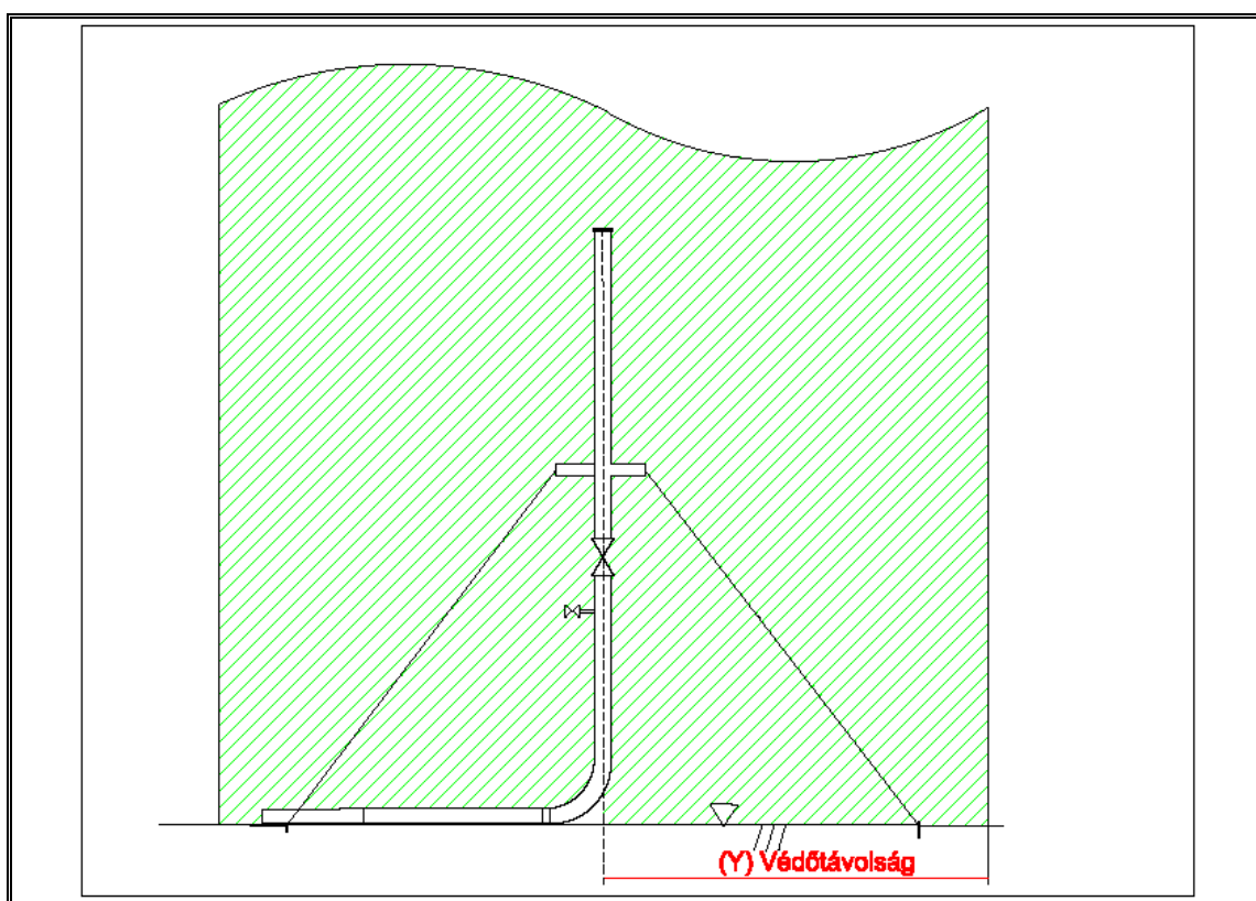
Védőtávolság kijelölésének módja 3.3.67. ábra
