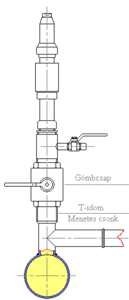
Acélcső nyomás alatti megfúró berendezés 3.3.80. ábra
