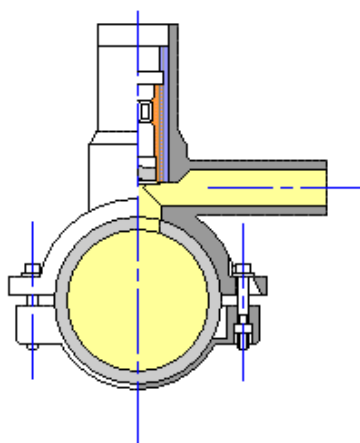
PE elektrofúziós megfúróidom 3.3.82 ábra
