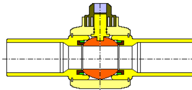
Hegtoldatos gömbcsap minta ábra (FRIALEN)
