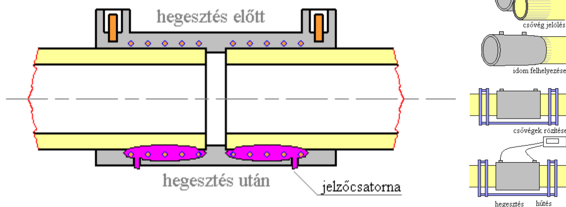
I.94 ábra Fűtőszálas tokos hegesztési varrat
