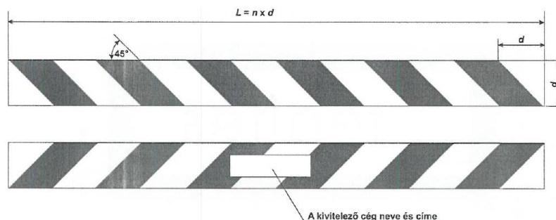
Az útelzáró korlát kialakítása
