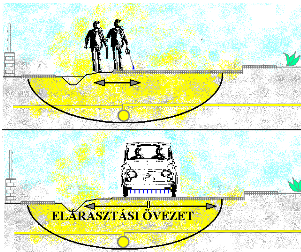
Tömörségellenőrzés alkalmazhatósági tartománya
