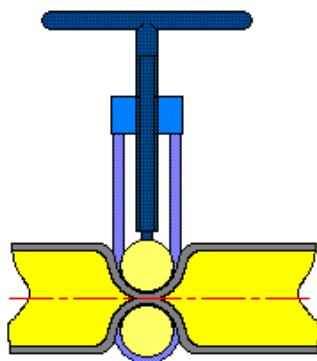
PE cső elszorítása csavarorsós elszorító-szerszámmal 3.3.77. ábra
