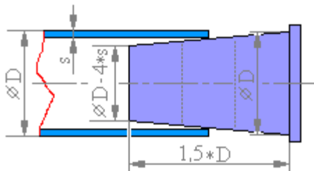
I.88. ábra Acél csővég kalibrálása
