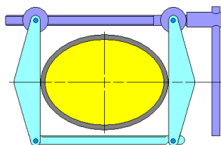
PE cső visszakerekítése elszorítás után 3.3.78. ábra
