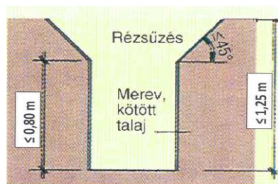
3.2.36 ábra Munkaárok kialakítása dúcolás nélkül
