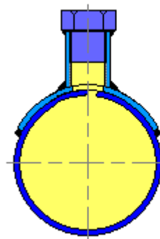
Acélkarmantyú 3.3.86. ábra
