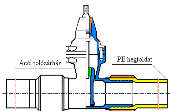
Fémházas tolózár polietilén csatlakozással minta ábra (AVK)
