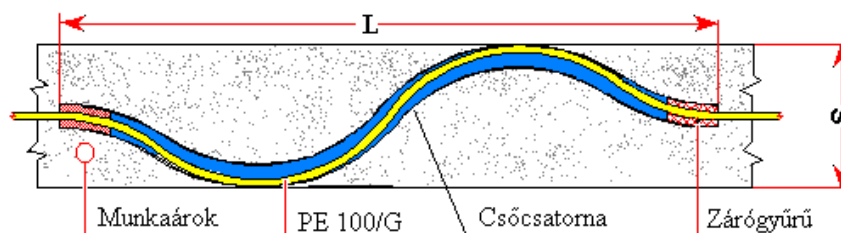
S – kompenzátor
