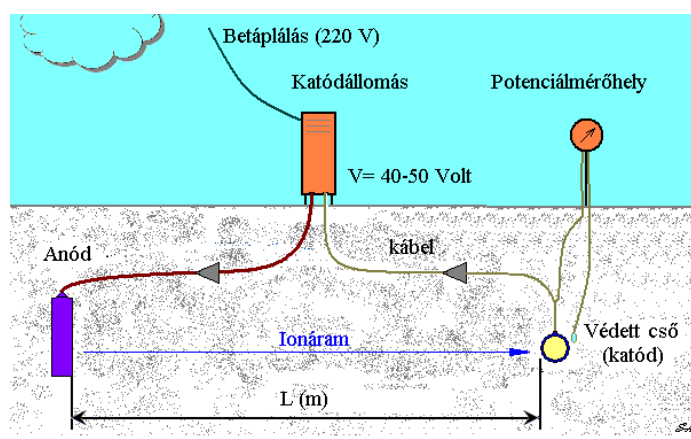
Külső áramforrással táplált katódos védelem 3.2.48 ábra
