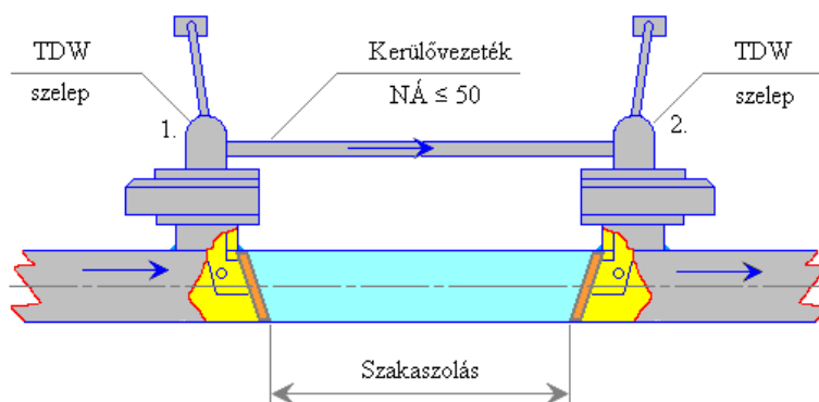
3.3.79 TDW szakaszoló-berendezés (elvi ábra)
