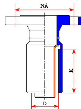
3.1.15. ábra Karimás PE-acél összekötő
