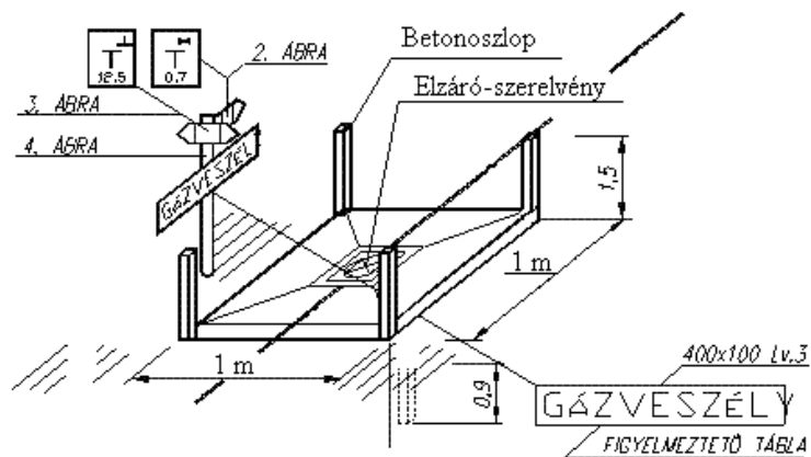
Külterületi szakaszoló elzáró védelme és jelölése
