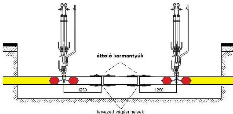
Gépi ballonozó berendezéssel kiszakaszolt vezeték 3.3.73. ábra
