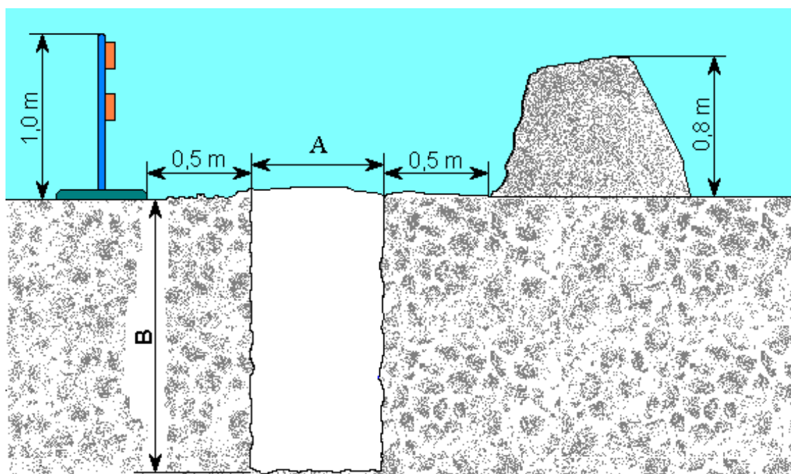
Munkaárok kialakítása, mérete
