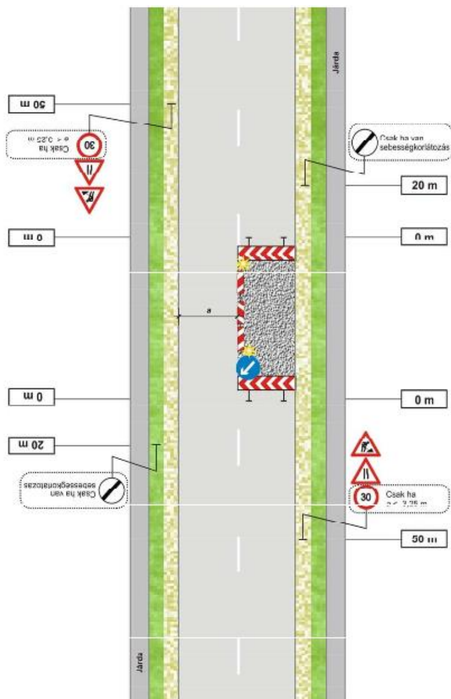
V.106 ábra Egy forgalmi sáv lezárása kisforgalmú úton (belterület)
