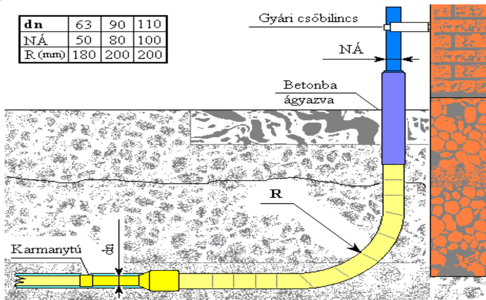
F4 jelű végpont 3.1.30 ábra
