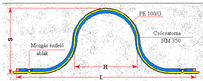
OMEGA – kompenzátor
