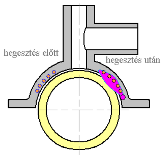
I.95 ábra Fűtőszálas nyereghegesztési varrat
