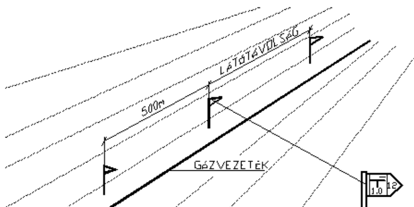
Jelzőoszlop beültetése egyenes csőszakaszon 3.2.61 ábra
