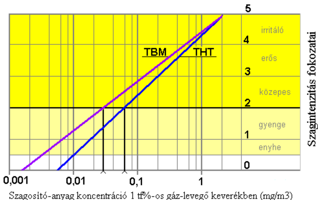
Szagintenzitás a szagosító-anyag koncentráció függvényében 3.3.65. ábra
