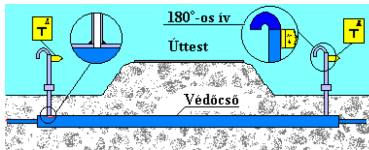
Nagy terhelésű védőcső-szagló jelölése jelzőzászlóval
