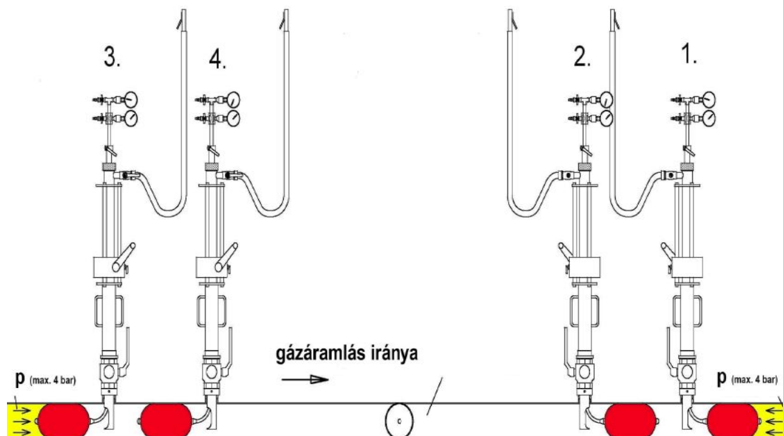
4 bar-os gépi ballonozó berendezéssel kiszakaszolt vezeték 3.3.74. ábra
