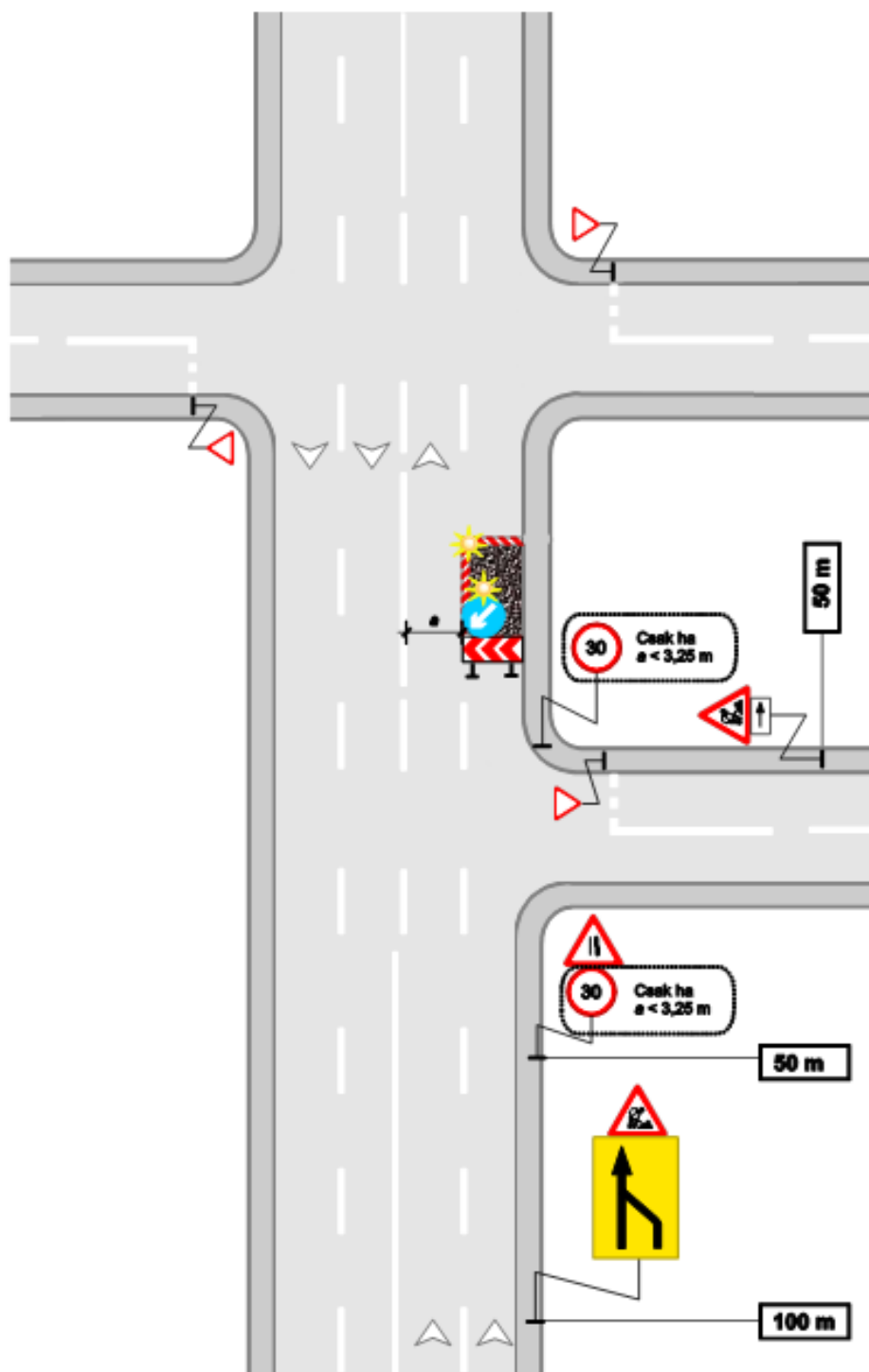
V.107 ábra Külső forgalmi sáv lezárása (belterület)
