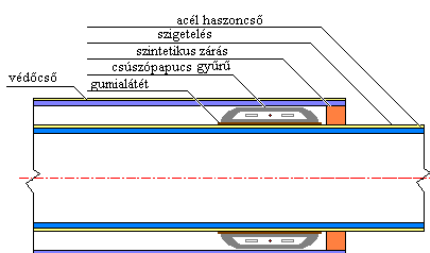
Acélcső védőcsőbe helyezése csúszógyűrűkkel
