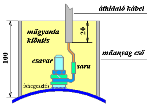
Fémes áthidalókötés 3.2.46 ábra
