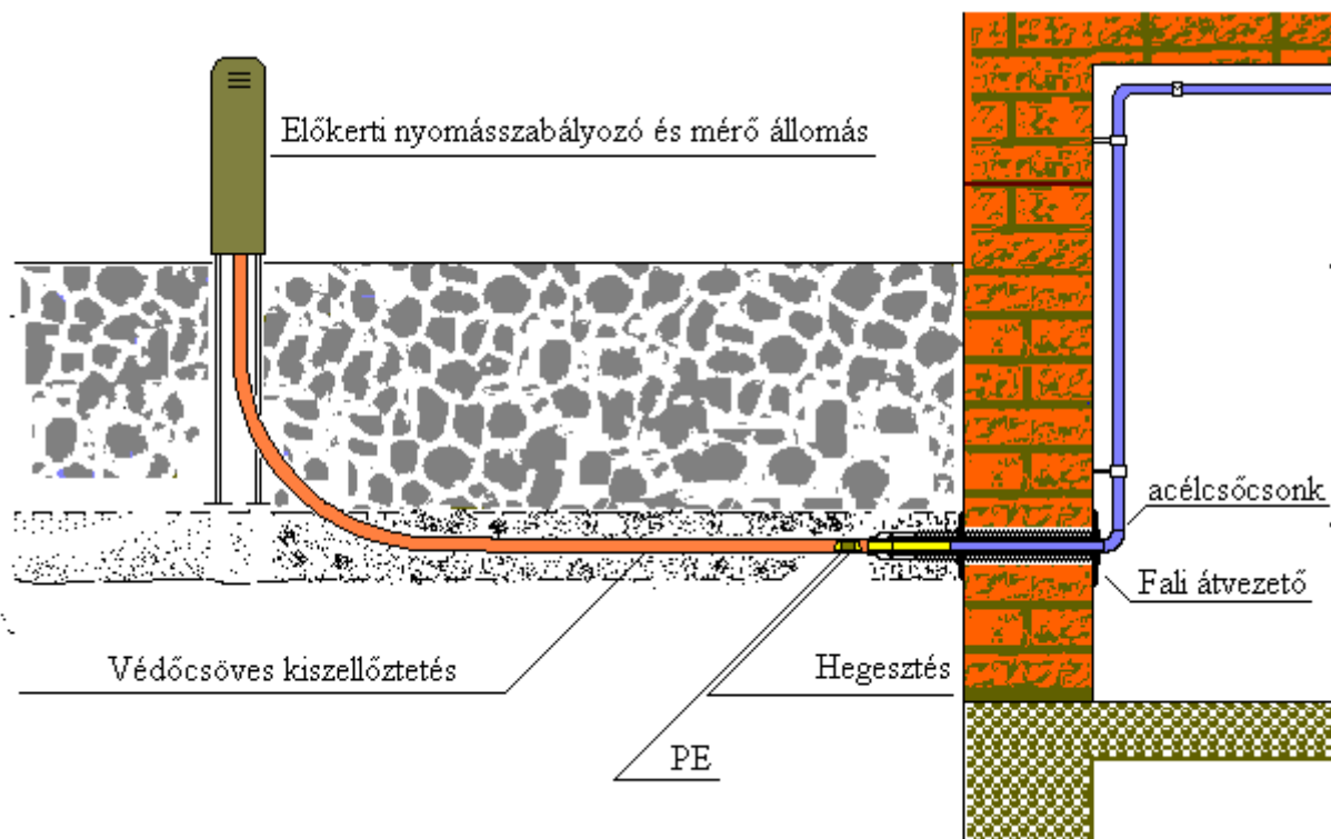
Pincei bevezető beépítési vázlata 3.1.23 ábra
