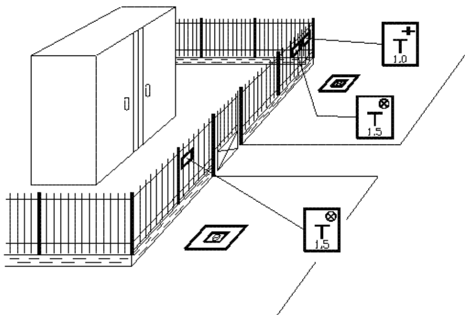
Nomásszabályozó állomás előtti vezetéki elemek jelölése
