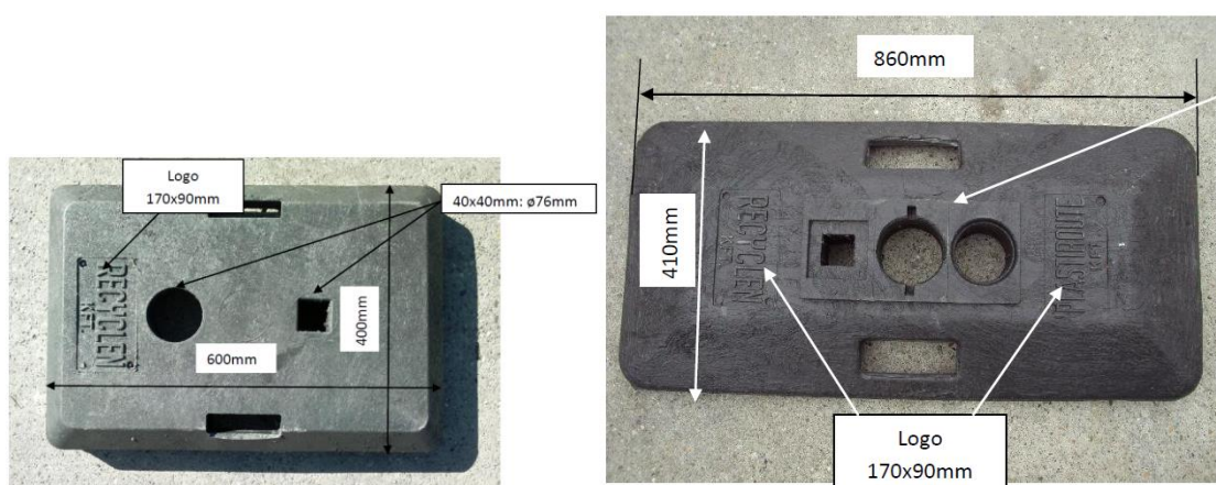
V.109 ábra ábra 20 és 28 kg-os műanyag leterhelő talpak
