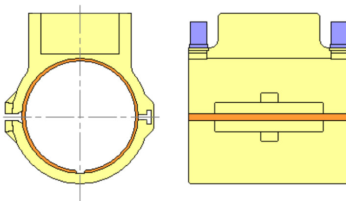
PE javító-lezáró idom 3.3.87. ábra
