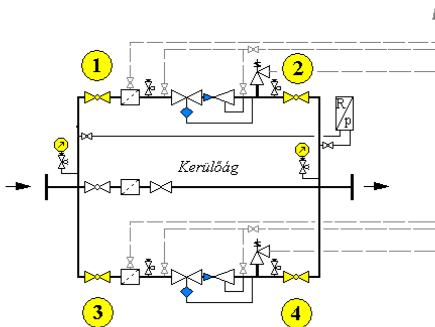
Egyágas nyomásszabályozó állomás leállítása III.-2.3 ábra
