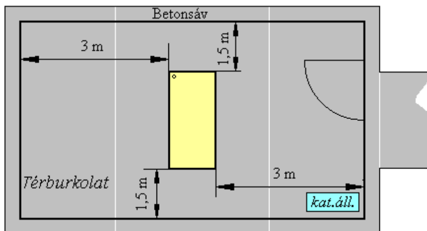
Nyomásszabályozó állomás területi kialakítása
